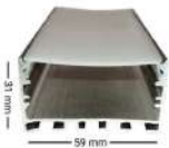
TS18R Power : 30W / 60W Color : White / Black Light : 6000K.4000K.3000K
