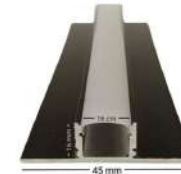
TS47 Power : 20W / 24W / 30W Color : White / Black Light : 6000K.4000K.3000K
